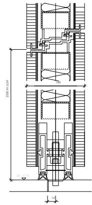
Türenelement
